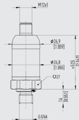
Con connettore circolare M12 x 1 (4 pin, metallico)
